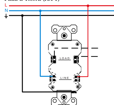
Toma de corriente dúplex Falla a Tierra (ICFT)
